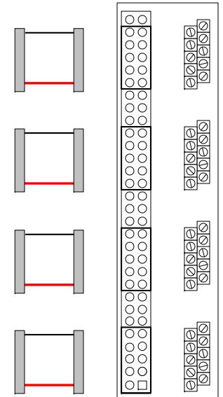
TB-10/10/10/10 CONFIGURATION
